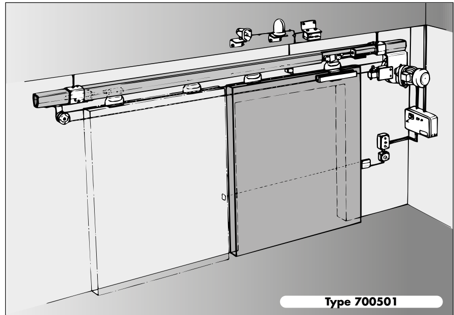
Fire protection sliding door with a DICTAMAT 700
