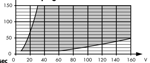
kg Damping force ÖDR 14-35
