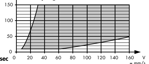
Kg Damping force ÖDR 14-35
