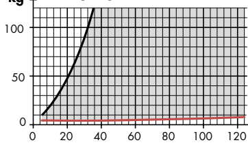
kg Damping force ÖDR 10-28
