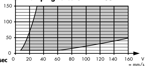
kg Damping force ÖDR 14-35
