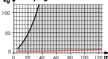
kg Damping force ÖDR 10-28
